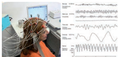
Abb. 6: Elektroenzephalografie
